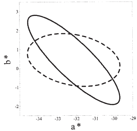
(d) CIE Green color center
